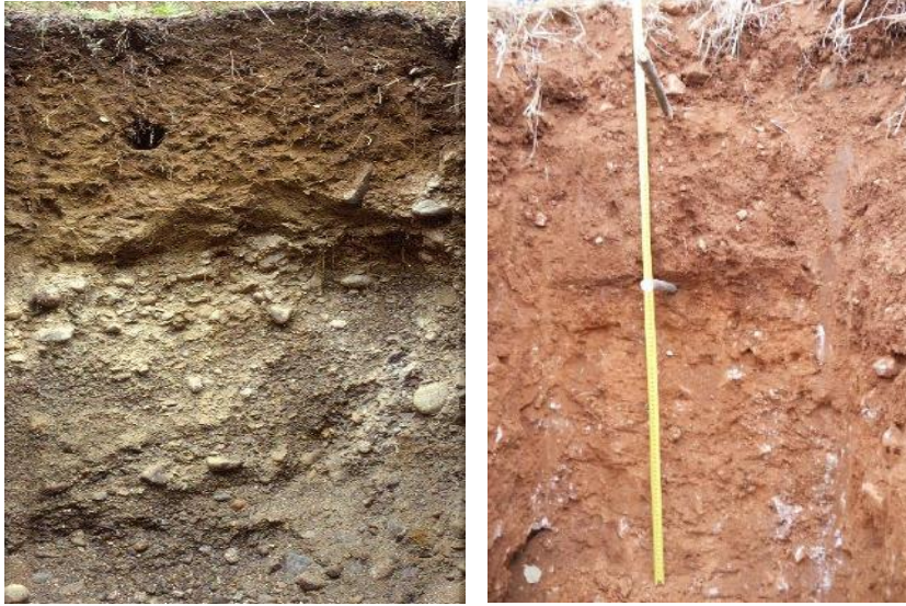
Şekil 2.5. Toprak Profilinin ve Solum (genetik toprak gövdesi) nin Farklı Görünümleri
