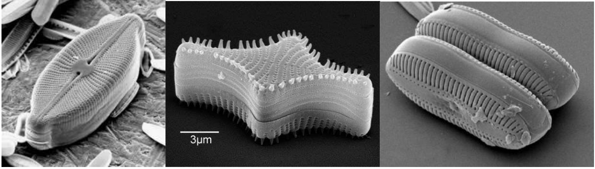
Şekil 4. Pennat diyatomeler
