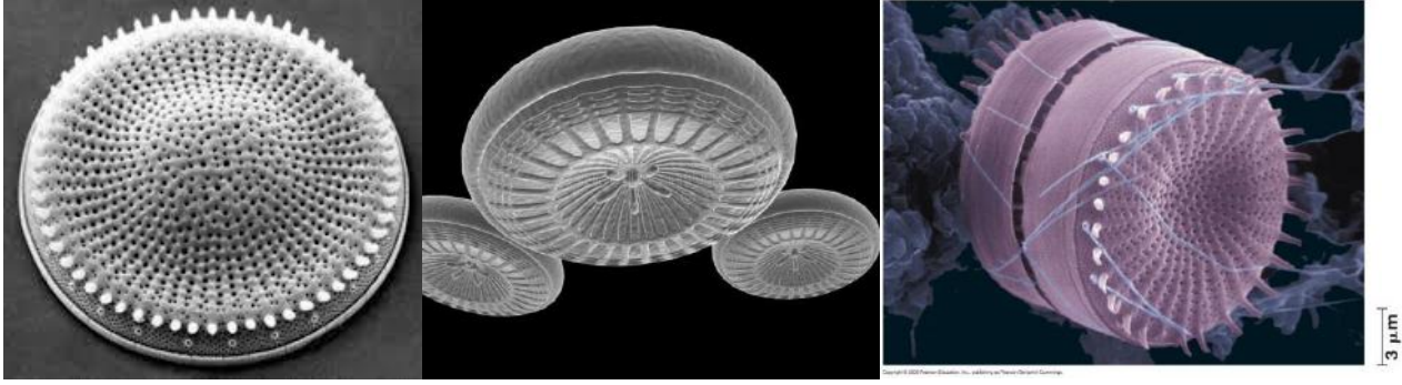
Şekil 3. Sentrik diyatomeler
